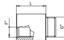
1530 Prelungitor M/F
