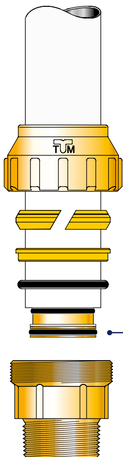
Art. 1476 Stut cu garnituri pentru tub multistrat (obligatoriu)
