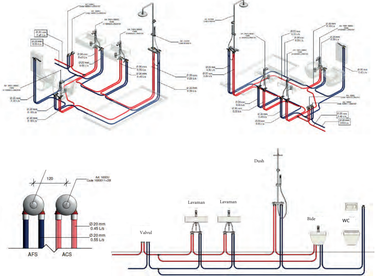
Shëmbul instalimi banjo me kolektor të paramontuar SANIBOX 3023 dhe 1481-1656
