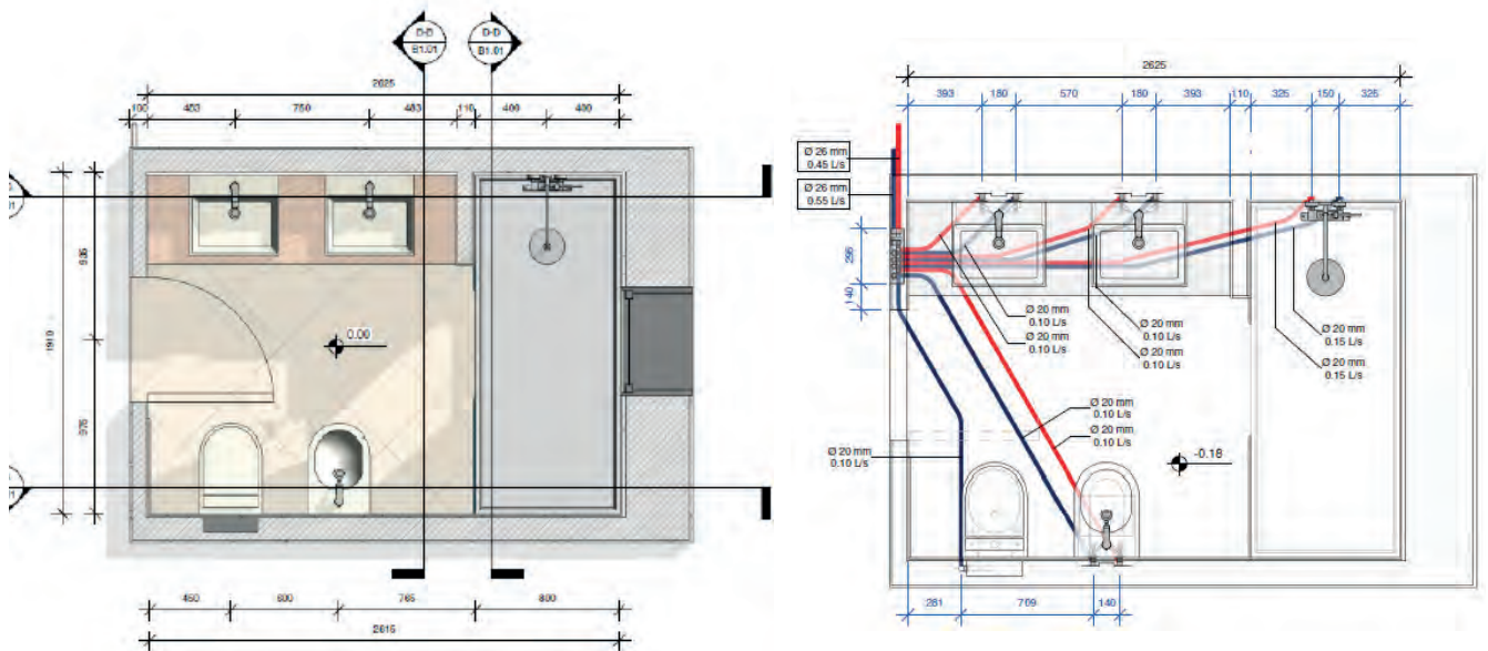
Shëmbul instalimi banjo me kolektor të paramontuar SANIBOX 3023 dhe 1481-1656
